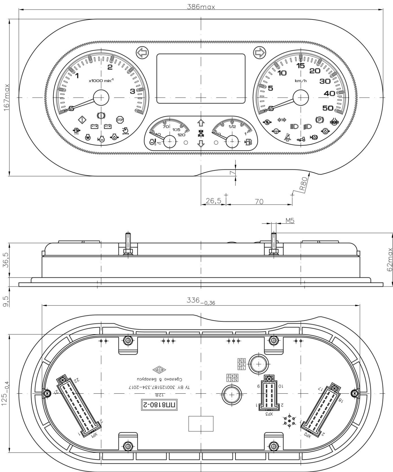
Рисунок А.2 - Габаритные и присоединительные размеры ПП-2
