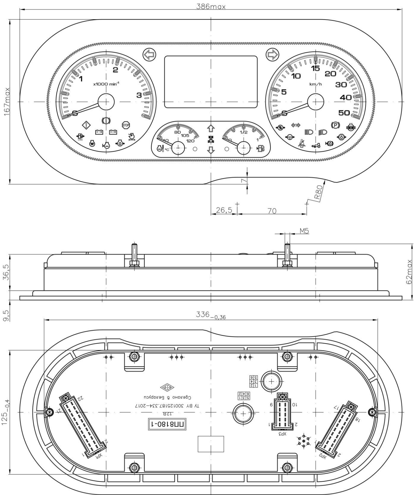
Рисунок А.1 - Габаритные и присоединительные размеры ПП-1
