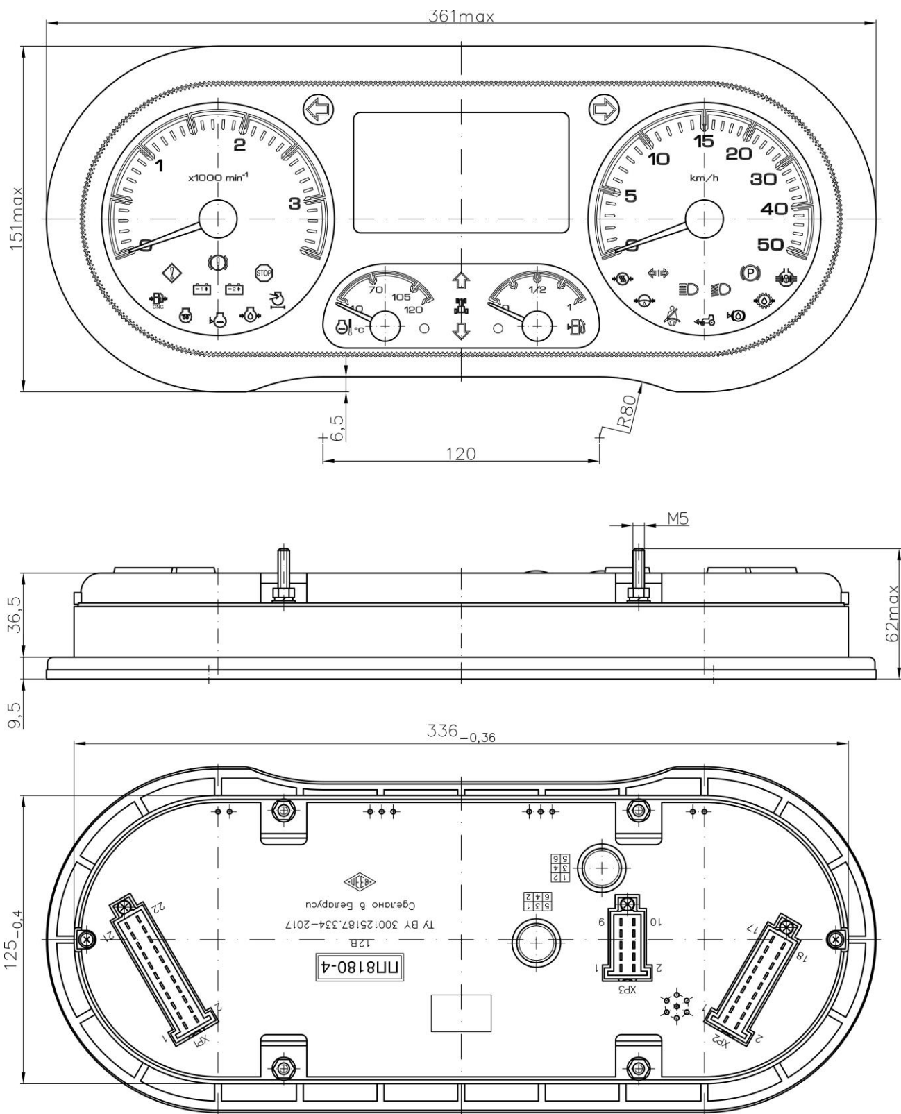
Рисунок А.4 - Габаритные и присоединительные размеры ПП-4
