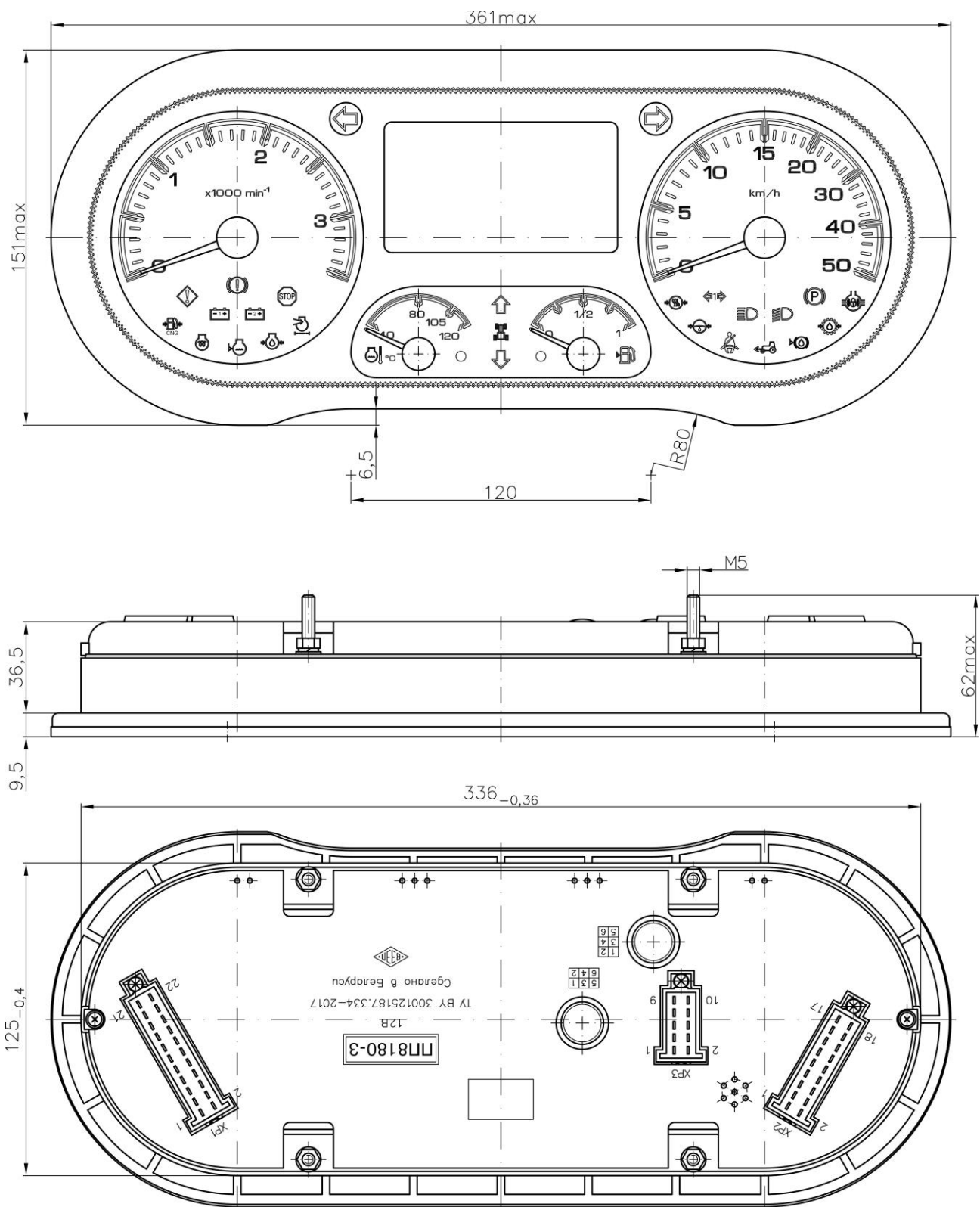
Рисунок А.3 Габаритные и присоединительные размеры ПП-3
